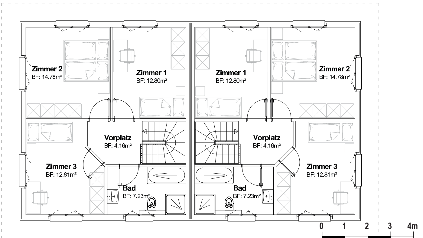
Obergeschoss 1:100
